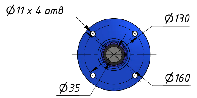
A-A (1:5)
